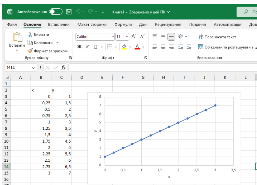
Рисунок 1.8 – Побудова відрізка
