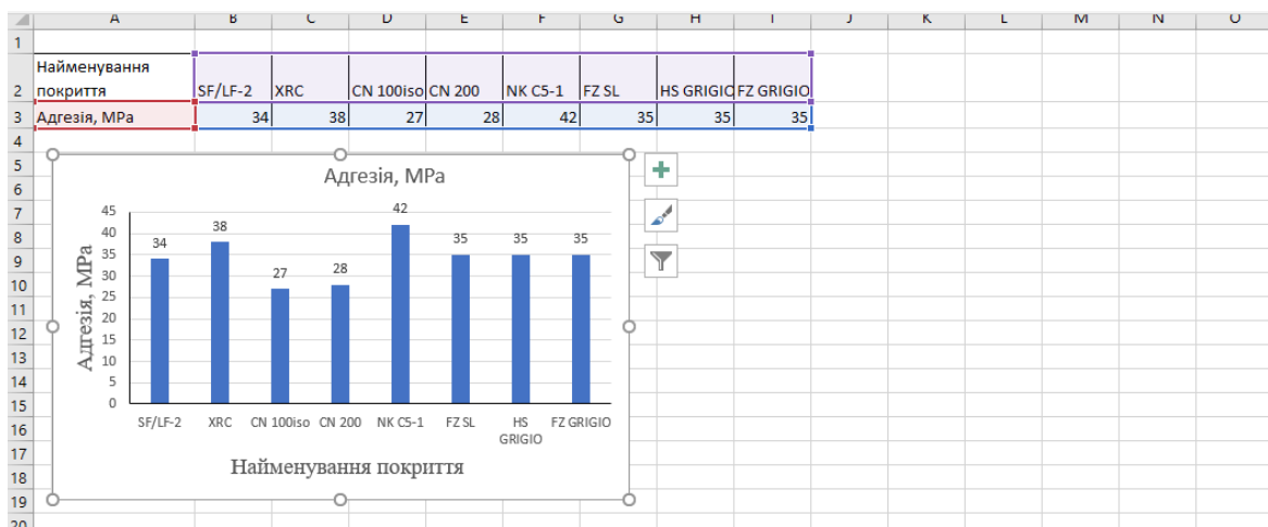
Рисунок 1.9 – Побудова гістограми
