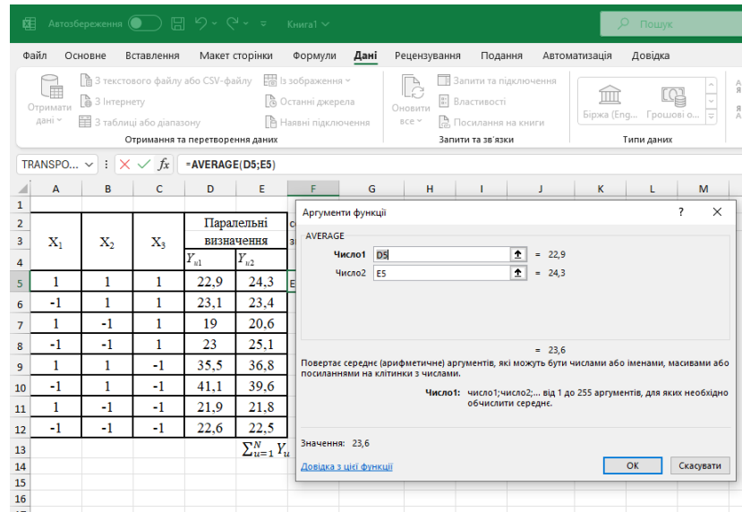
Рисунок 4.1 – Розрахунок дисперсії
